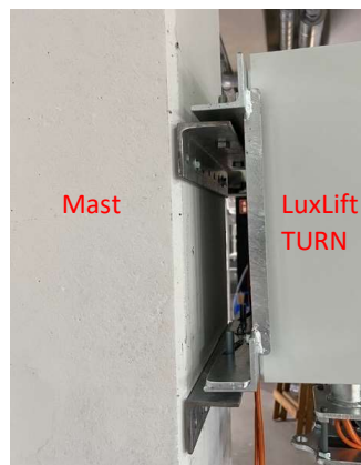
Einhängung des LuxLift TURN
