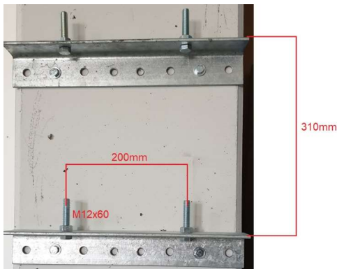
Befestigung der Montagebügel an den Mast
