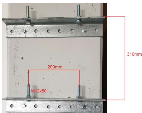
Upevnenie montážnych konzol na stĺp
