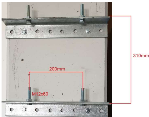
Szerelőkonzolok rögzítése az oszlophoz
