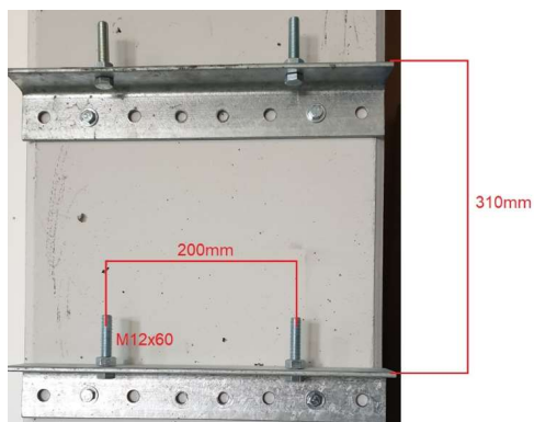
Pričvršćivanje montažnih nosača na stup
