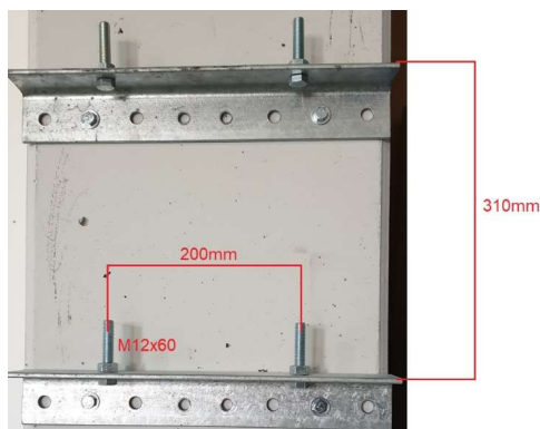
Upevnění montážních konzol na sloup
